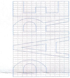
DETALHE PINTURA DE PARE Tinta: EXTRUDADO Cor: BRANCA ESPECIFICAÇÕES: MEDIDAS: COMPRIMENTO=1,35m ALTURA DA LEGENDA=1,00m
