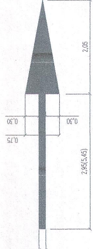
DETALHE DE SETA DE SENTIDO DE TRÁFEGO Tinta: EXTRUDADO Cor: BRANCA
