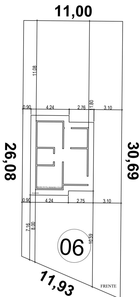
IMPLANTAÇÃO PADRÃO 02 QUADRA 8 LOTE 06
