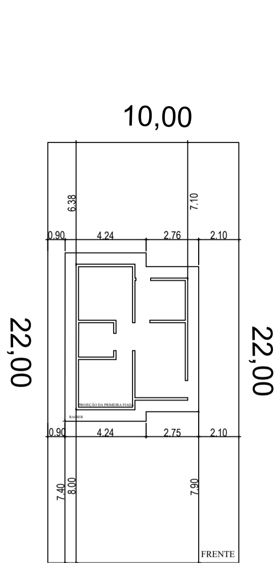
IMPLANTAÇÃO PADRÃO 01 QUADRA 8 LOTES 01 A 05 QUADRA 8 LOTES 10 E 11 QUADRA 11 LOTES 01 A 08 QUADRA 11 LOTES 13 A 19
