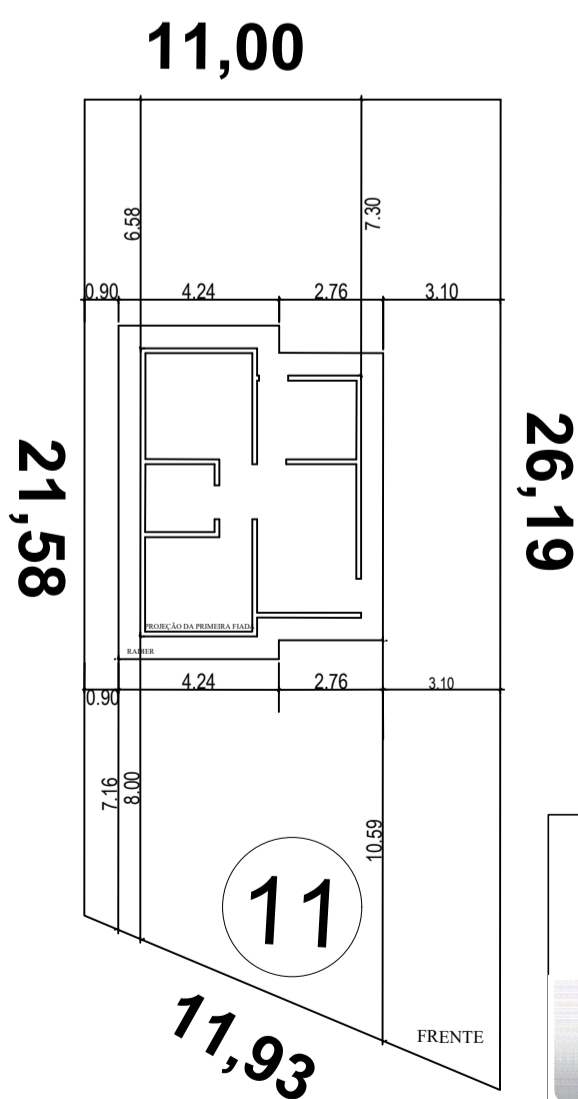
IMPLANTAÇÃO PADRÃO 07 QUADRA 11 LOTE 11
