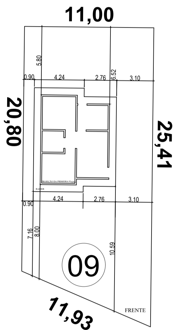
IMPLANTAÇÃO PADRÃO 05 QUADRA 11 LOTE 09
