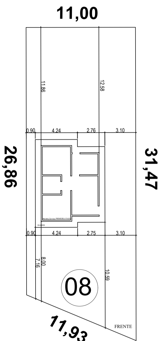
IMPLANTAÇÃO PADRÃO 03 QUADRA 8 LOTE 09
