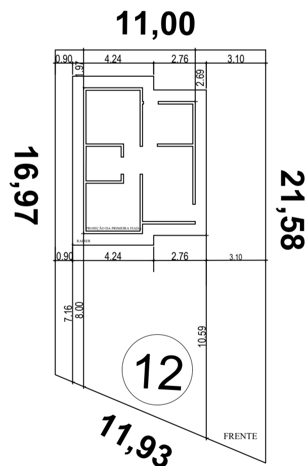
IMPLANTAÇÃO PADRÃO 08 QUADRA 11 LOTE 12
