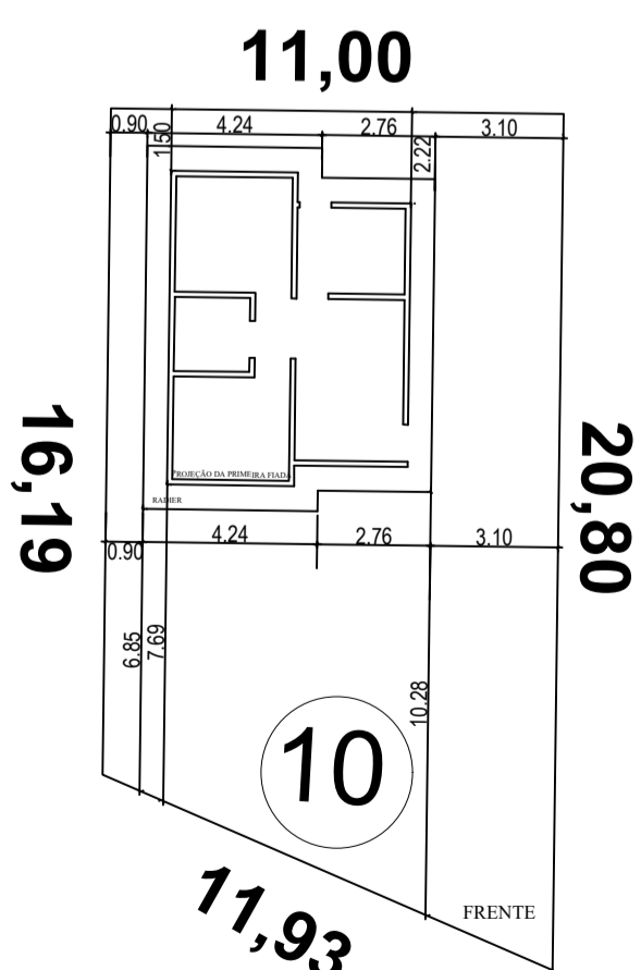
IMPLANTAÇÃO PADRÃO 06 QUADRA 11 LOTE 10
