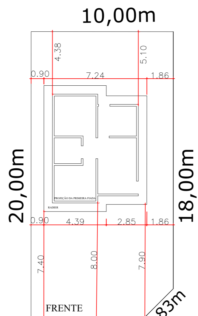
10,00m 20,00m 10,00m IMPLANTAÇÃO PADRÃO 02 QUADRA 01 - LOTE 03 QUADRA 02 - LOTE 32
