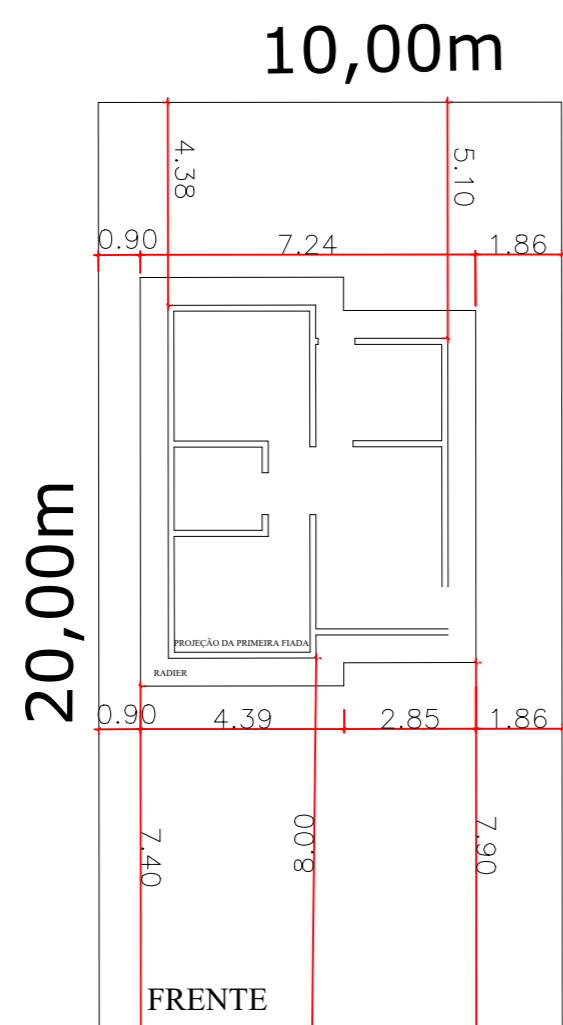
10,00m 20,00m 10,00m IMPLANTAÇÃO PADRÃO 01 QUADRA 01 - LOTES 02 AO 16 QUADRA 02 - LOTES 02 AO 14 QUADRA 02 - LOTES 19 AO 31 QUADRA 02 - LOTES 33 AO 34
