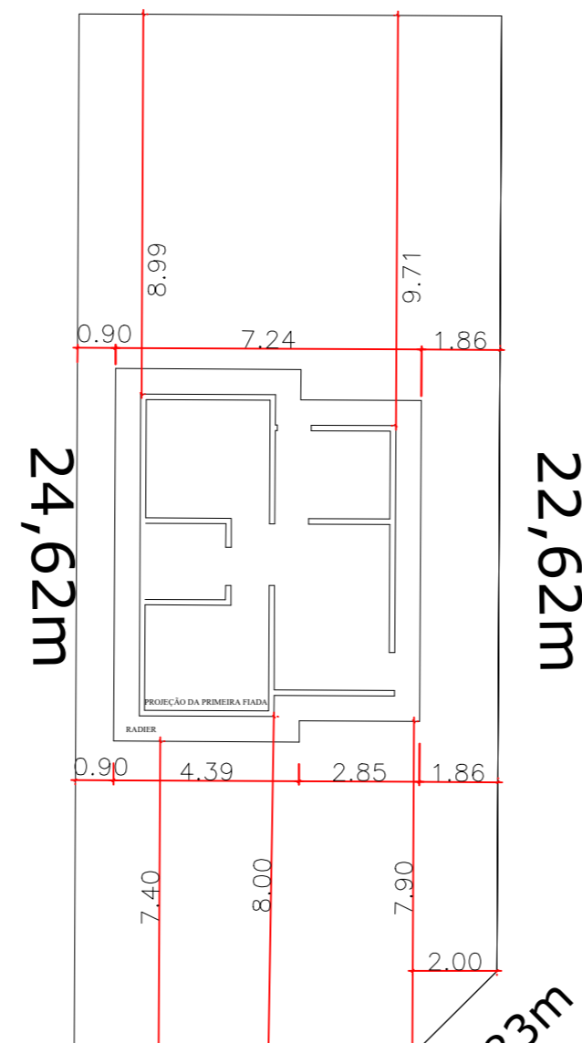
10,00m 22,62m 8,00m IMPLANTAÇÃO PADRÃO 06 QUADRA 02 - LOTE 15
