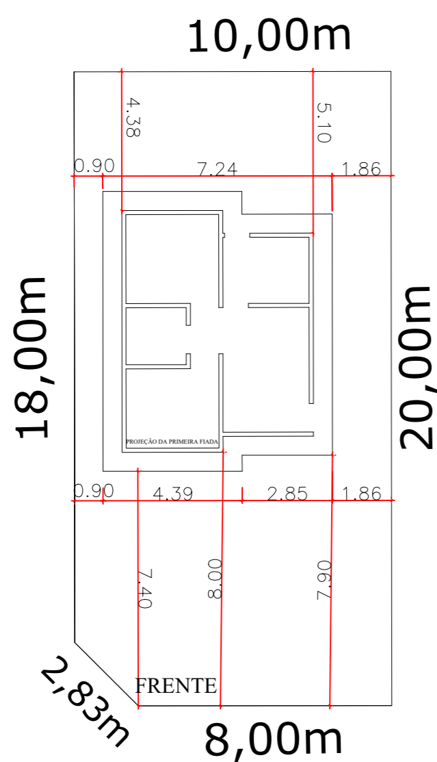
10,00m 18,00m 8,00m IMPLANTAÇÃO PADRÃO 05 QUADRA 02 - LOTE 01
