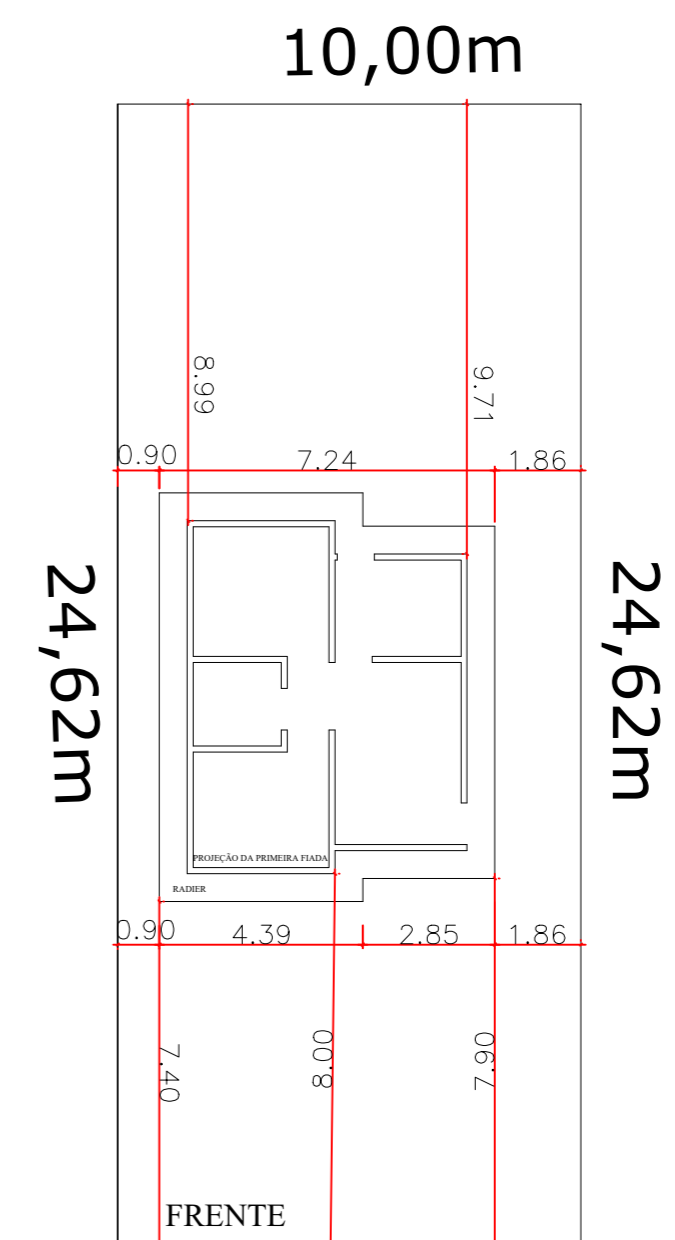
10,00m 24,62m 10,00m IMPLANTAÇÃO PADRÃO 04 QUADRA 01 - LOTE 18 QUADRA 02 - LOTES 16 E 17
