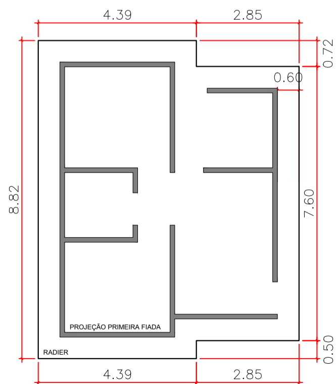
DETALHE - RADIER ESC. 1/100
